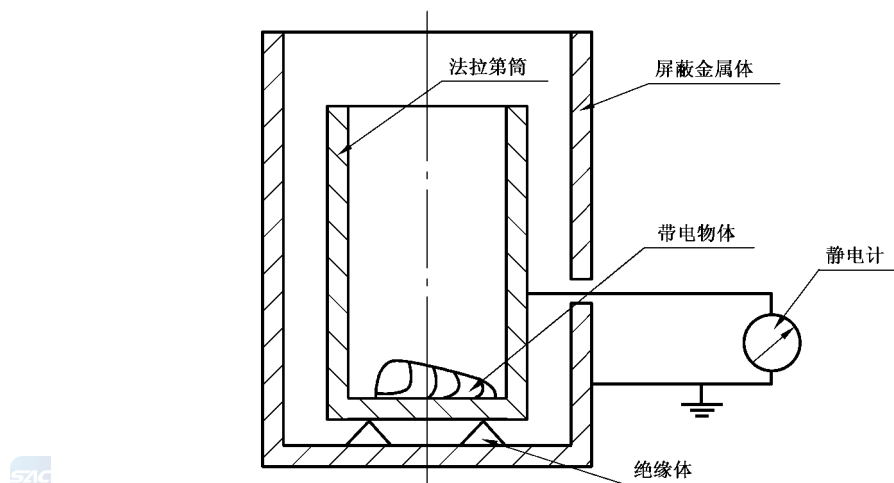
图 A.1 法拉第筒法原理图
